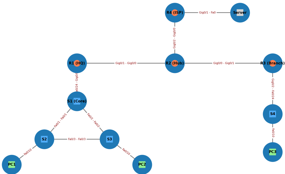
Logička Mrežna Topologija: Centrala i Filijala (Hub & Spoke)
